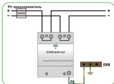
V-подключение ограничителя ETITEC B-PV
