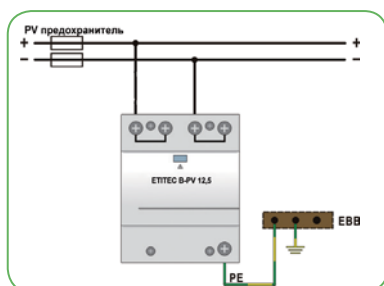
Т-подключение ограничителя ETITEC B-PV
